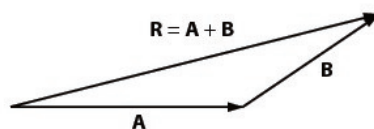
■ Gambar 1.4 Penjumlahan Dua Buah Vektor
